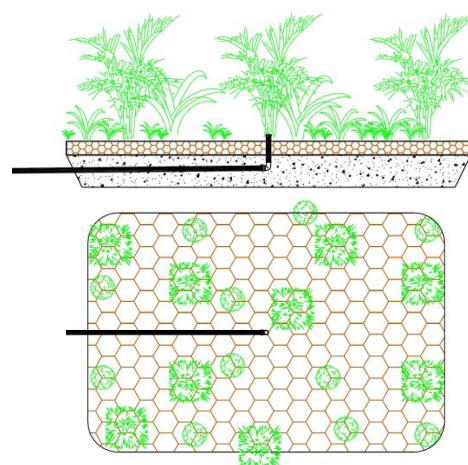
Schemat budowy poletka roślinnego
